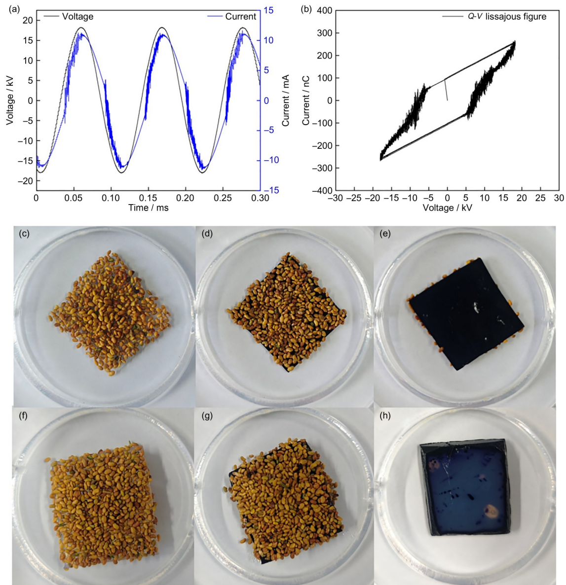
图2 电压-电流波形图与活性粒子显色评估
