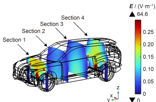
图8 车厢内不同位置感应电场强度沿不同XZ截面分布 along various XZ sections
