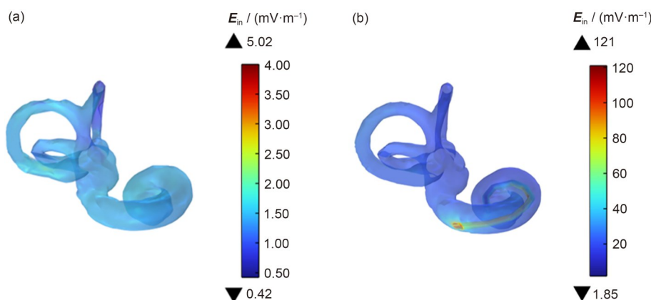
图9 内耳 E_m 分布:(a)普通乘客;(b)佩戴人工耳蜗乘客
