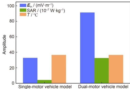
图 13 不同车型内乘客内耳暴露水平对比
